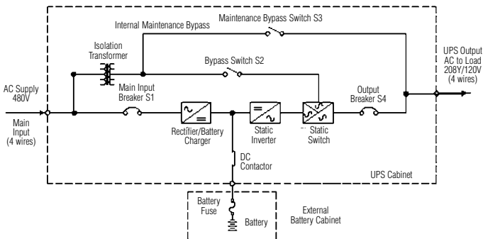
30 kVA (4 x 2)
