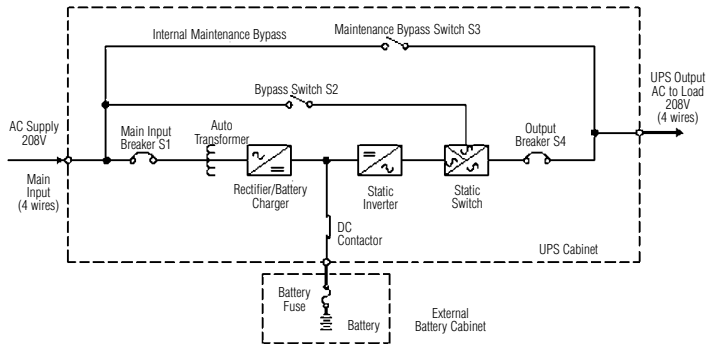
30 kVA (2 x 2)
